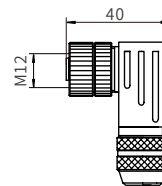
五针90° 航插母头
