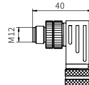
五针90° 航插公头
