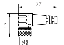
四针90° 航插母头
